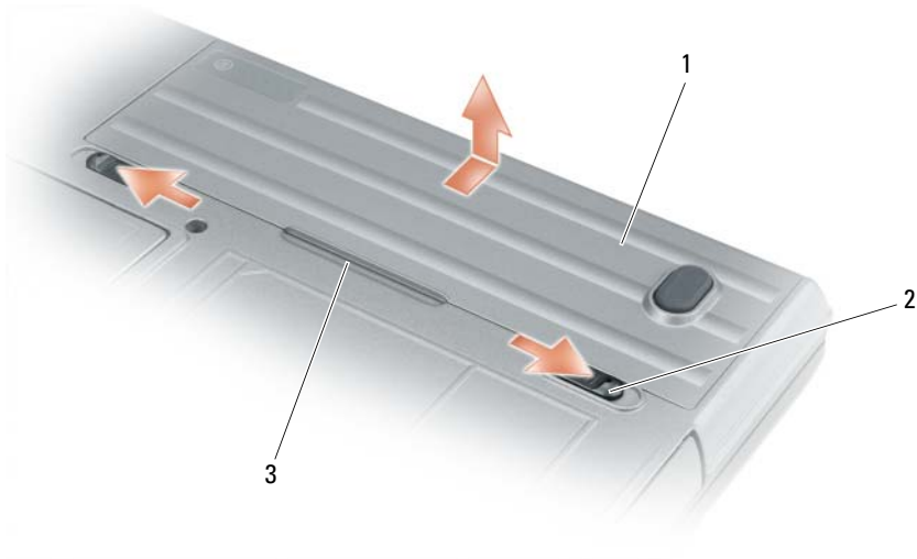
1 电池 2 电池槽释放闩锁 (2) 3 电池卡舌
